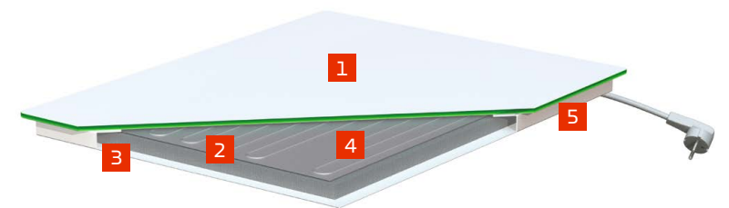
Schnittbild Vitoplanar Infrarotheizung
